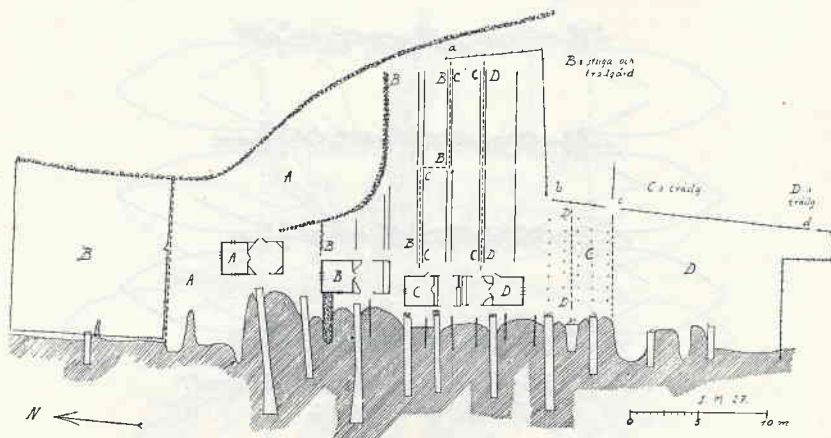
Fig. 94. Båtkåser och sjöbodgårdar. Småland.
