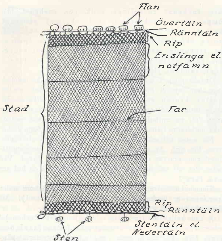
Fig. 81. Ett telnskott i notarm. Uppland.
