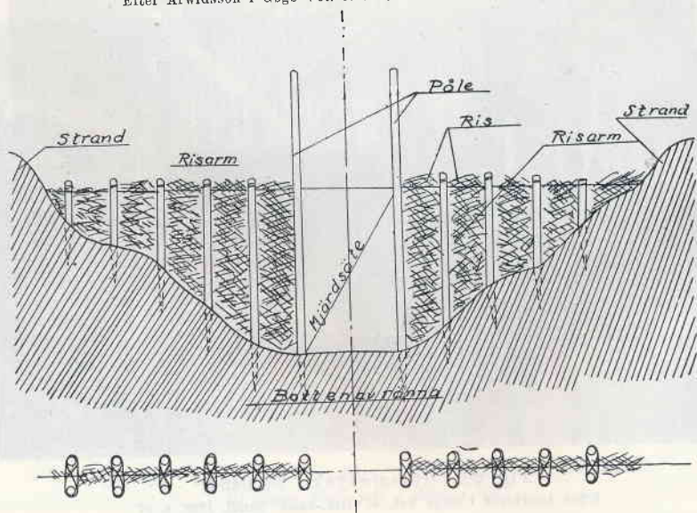
Fig. 30. Mjärdsäte med risarmar. Dalarna. Ur Nord. mus. arkiv, Etnol. undersökn. 3369, s. 2.
