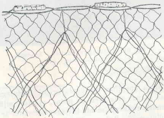
Fig. 62. Skottnät. Hälsingland. Ur Ekman Norrl. jakt och fiske, s. 312.
