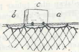
Fig. 60. Skjutning av sillgarn, detalj. Skåne.
