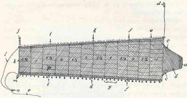
Fig. 79. Vinternot, ena armen och kilen. Uppland.
