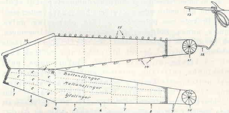
Fig. 80. Landnot med »bågar», en tög och »notkrycka».
