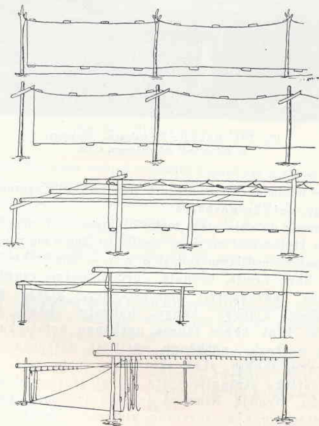
Fig. 99. Torkställningar för nät.
