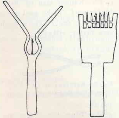
Fig. 5. Ålegil (av olika typer). Bohuslän.
