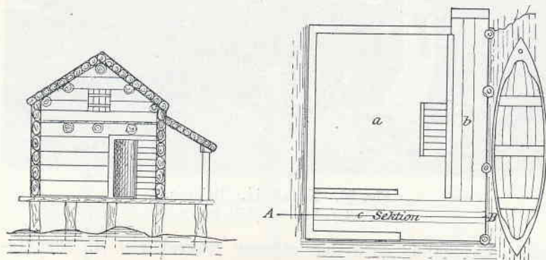
Fig. 95. Sjöbod med svale. Hälsingland. Ur Svenska landsmål 1913, s. 7 (fig. 1, 2).
